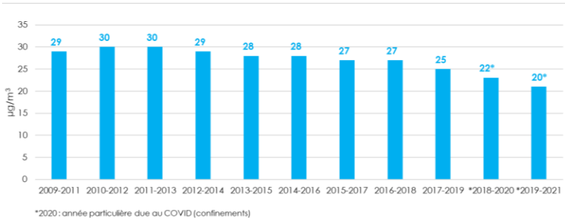
Évolution de la concentration moyenne 3 ans en NO 2 sur la station de fond de l'Essonne (Evry)
