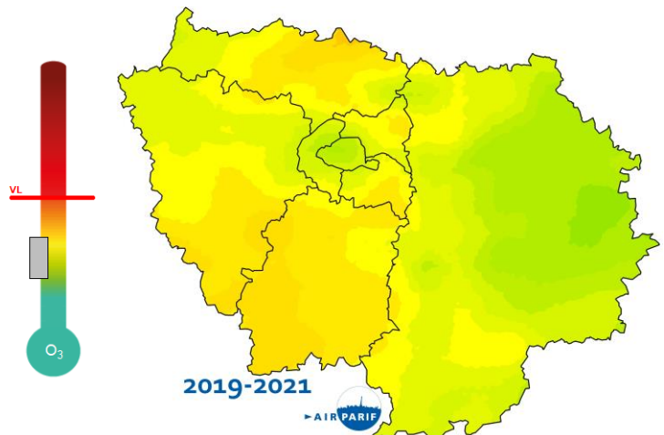
Situation de l'Île-de-France au regard de la valeur cible en ozone pour la santé (seuil de 120 µg/m 3 sur 8 heures) – période 2019-2021.
